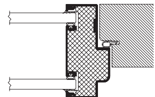
DEKO TD - Solid timber door
