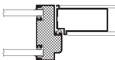
DEKO DG - Double glazed door
